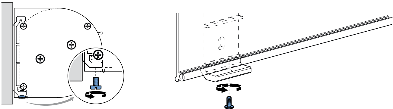
fig. 2.5 Aanbrengen vergrendelingsbouten
