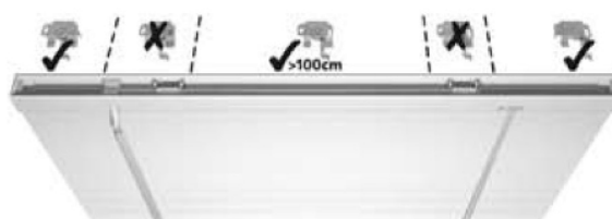
Plaatsing van de montagebeugels op de bovenbak.
